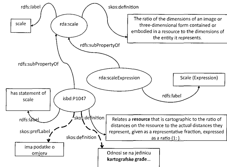
Slika 5.b Metoda A: primjena ISBD-a, pri čemu je za svojstvo definirana domena klasa – resurs (resource – kartografska građa), a hrvatski prijevod ISBD elemenata prikazan u imenskom prostoru ISBD elementa kao skos:prefLabel
