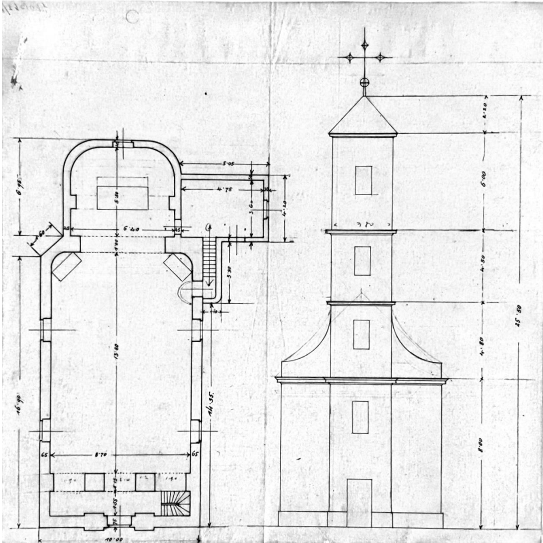
Slika 103: Nacrt crkve sv. Mateja u Garčinu iz Državnog arhiva u Slavenskom Brodu.
