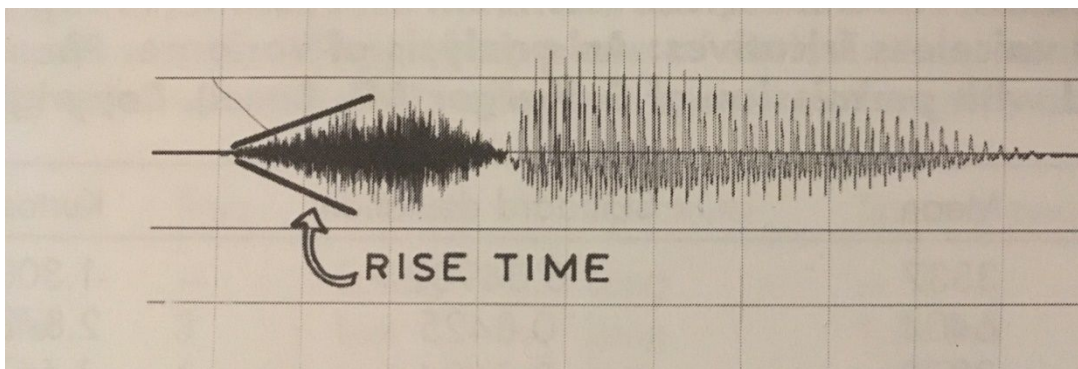
Slika 3. Oscilogram počeka riječi shoe (Kent i Read, 2002)
