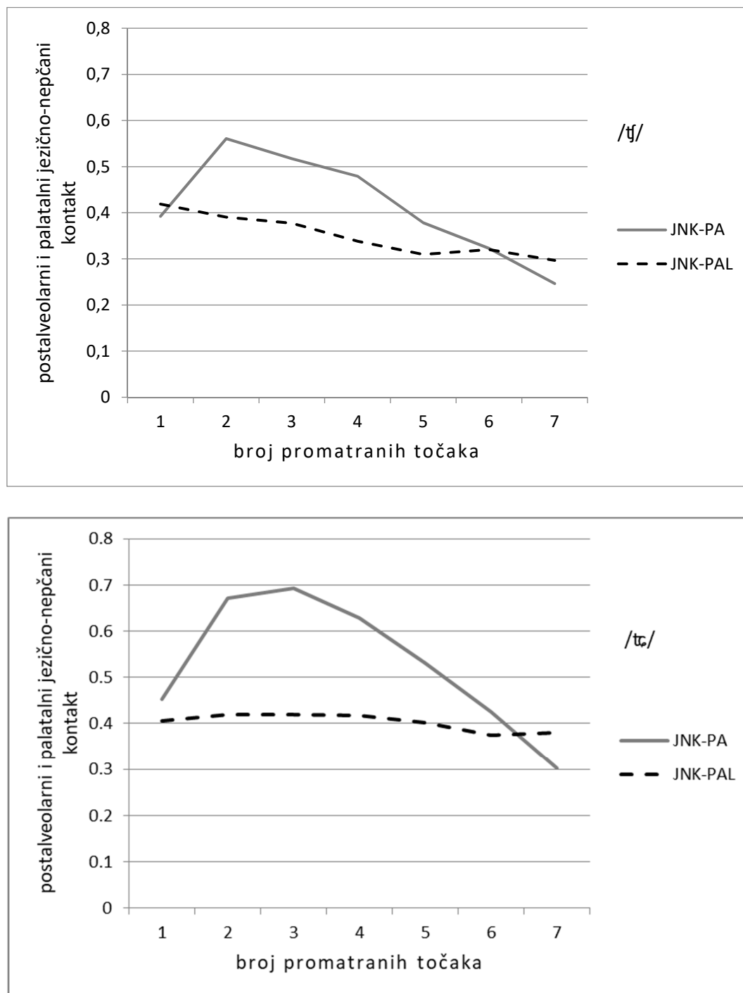
Slika 22. Prikaz uprosječenih mjera postalveolarnoga i palatalnoga jezično-nepčanoga kontakta ispitanice I5 za afrikate /č/ i /č̟/
