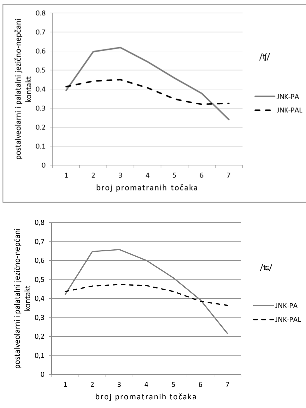
Slika 21. Prikaz uprosječenih mjera postalveolarnoga i palatalnoga jezično-nepčanoga kontakta ispitanice I4 za afrikate /č/ i /č̞/
