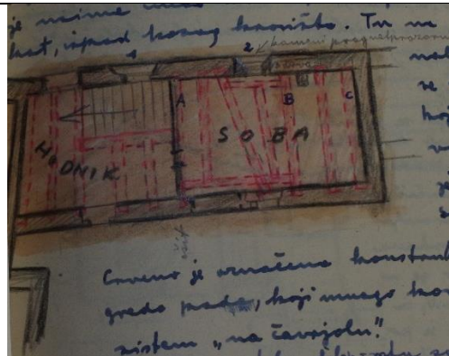
sl.26. Sustav greda na katu atrija i samostanske zgrade
