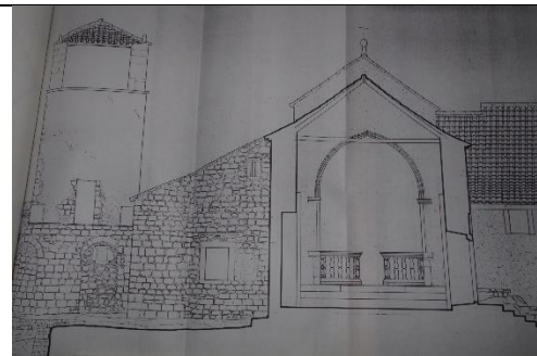
sl.36. Presjek – otvori na romaničkom trijemu
