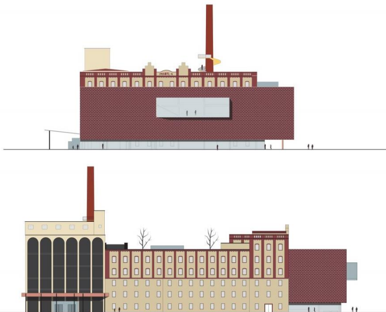
Sl. 33. Jana Čulek, natječajni projekt za novu Gradsku knjižnicu na lokaciji Paromlin, gore: pogled sa sjeverne strane, dolje: pogled sa istočne strane, Zagreb, 2019.
