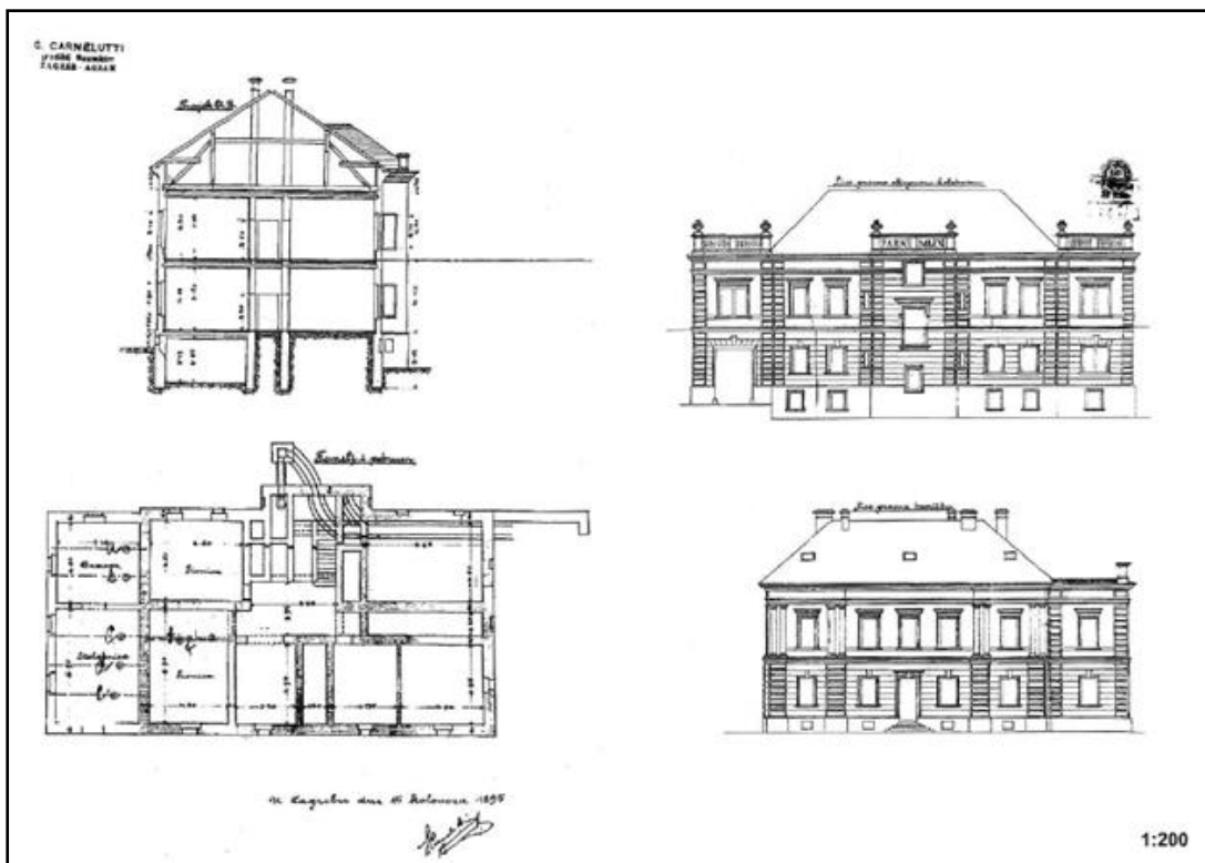
Sl. 8. G. Carnelutti, upravna zgrada, poprečni presjek a-b- i flocrta temelja i podruma (lijevo); pročelje prema glavnom kolodvoru i dvorišno pročelje (desno), 1985. godine
