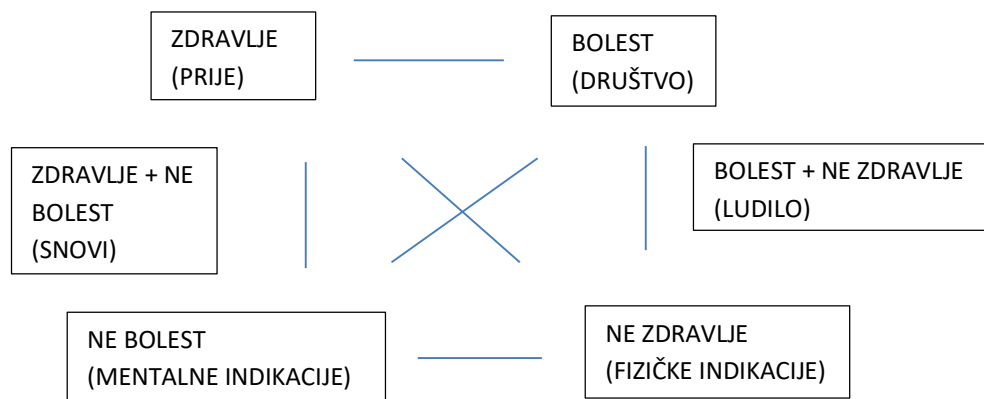
Slika 8. Semiotički kvadrat
