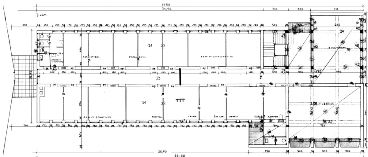
Slika 110. Tlocrt 1. kata Gradske uprave
