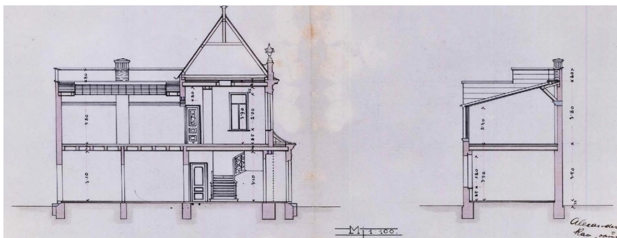
Sl. 33. Nacrt za fotografski atelijer u dvorištu kuće gosp. pl. Weissa, Ilica br. 8, prerez A–B i prerez C–D, 1894., Državni arhiv u Zagrebu
