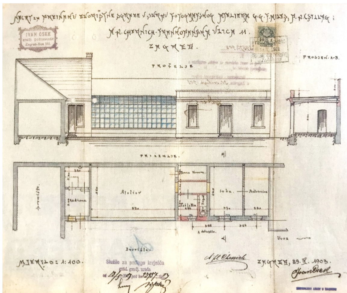
Sl. 52. Nacrt za preinaku dvorišne zgrade u svrhu fotografskog atelijera, Frankopanska ulica br. 11, 1903., repro: Slavko Šterk, Stereoskopska fotografija na prijelomu 19. u 20. stoljeće iz fundusa Muzeja grada Zagreba , katalog izložbe (Muzej grada Zagreba, studeni-prosinac 2002.), Zagreb: Muzej grada Zagreba, 2002., str. 26.
