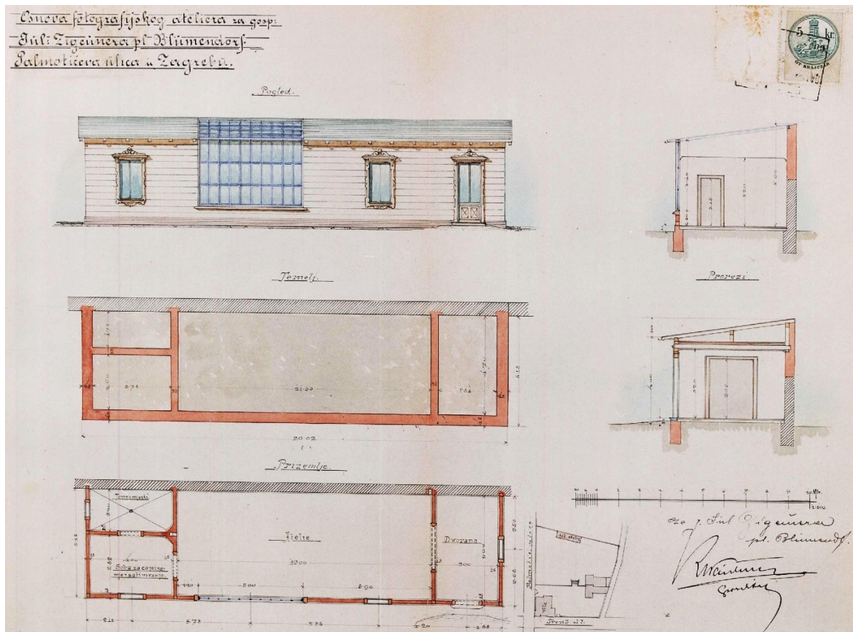
Sl. 39. Osnova fotografiskog atelijera za gosp. J. Zigeunera pl. Blümendorfa u Palmotičevoj ulici (ugao s Dordićevom ul.), 1892.; Izvor: HR-DAZG-866 Zbirka fotografija. AG 52
