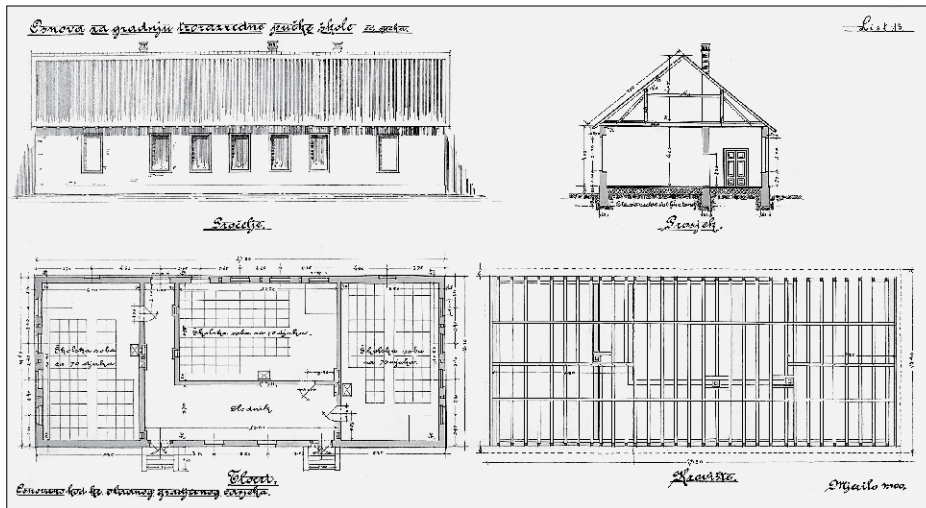
SL. 24. GRAĐEVNI ODSJEK ZEMALJSKE VLADE: TIPSKE PROJEKTI ZA IZGRADNJU TROSTRZREDNE PUČKE ŠKOLE U HRVATSKOJ, 1895.
