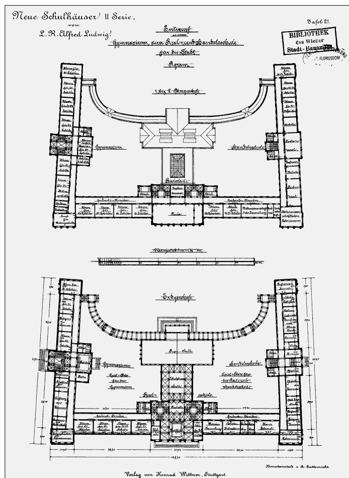
Sl. 6. LUDWIG & HÜLSSNER: PROJEKT ZA ZGRADU KRALJEVSKE VELIKE GIMNAZIJE, REALKE I TRGOVAČKE ŠKOLE U ZAGREBU, TLOCRTI, 1894.
