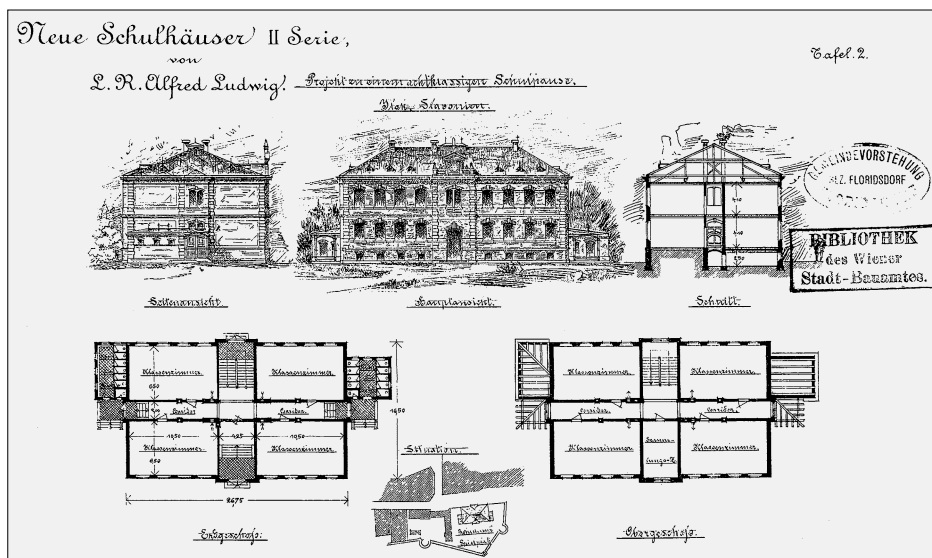
Sl. 20. LUDWIG & HÜLSSNER: PROJEKT ZA ZGRADU SKOLE S OSAM UČIONICA U ILOKU, 1894.
