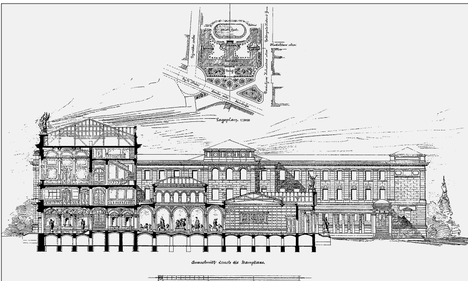
SL. 4. LUDWIG & HÜLSSNER: PROJEKT ZA ZGRADU KRALJEVSKE VELIKE GIMNAZIJE, REALKE I TRGOVAČKE SKOLE U ZAGREBU, PRESJEK, 1894.
