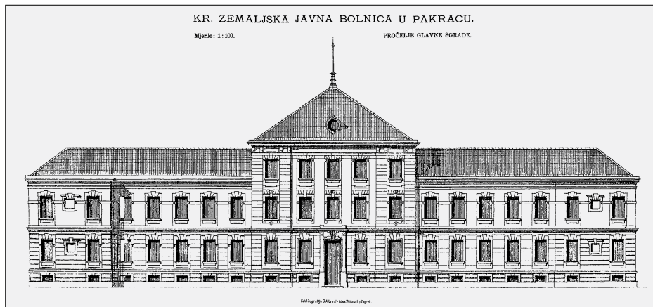
SL. 30. GRAĐEVNI ODSJEK ZEMALJSKE VLADE: IZVEDENI PROJEKT ZA GLAVNO PROČELJE SREĐIŠNJE ZGRADE KRALJEVSKE ZEMALJSKE JAVNE BOLNICE U PAKRACU, OKO 1896.
