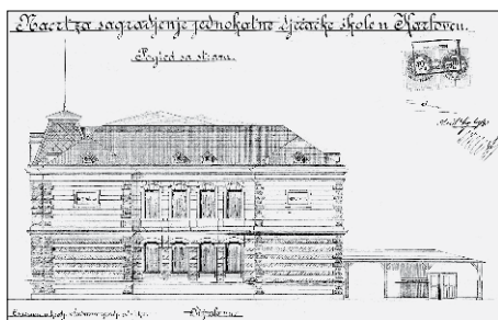
SL. 16. GRAĐEVNI ODSJEK ZEMALJSKE VLADE PREMA LUDWIGU & HÜLSSNERU: PROJEKT ZA BOČNO PROČELJE DJEČAČKE SKOLE U KARLOVCU, 1894.
