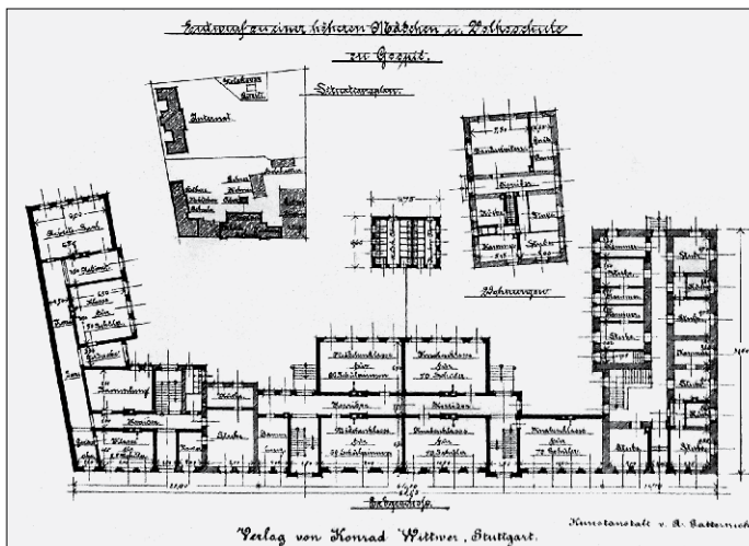
SL. 18. LUDWIG & HÜLSSNER: PROJEKT ZA ZGRADU DJEČACKE, DJEVOJAČKE I VIŠE DJEVOJAČKE ŠKOLE U GOSPIĆU, TLOCRTI 1894.
