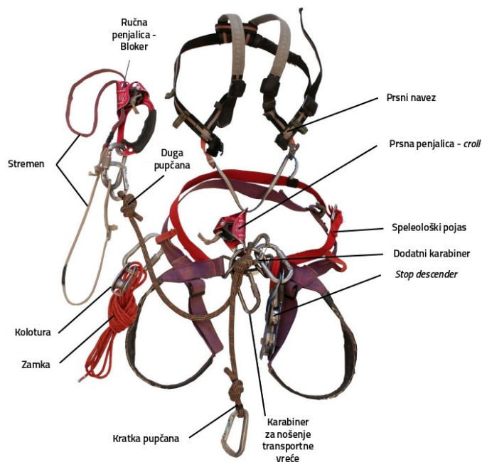
Slika 10.13 | Oprema speleologa za kretanje po užetu
