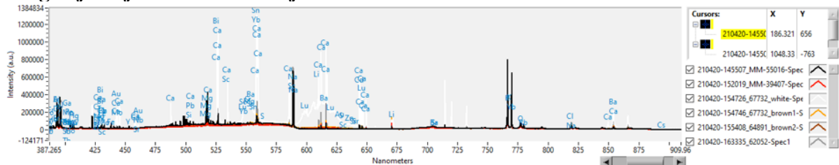
Tablica 8 Graf s prikazima Ca u bijelom premazu u usporedbi s premazima drugačije boje na helenističkoj keramici iz Ise
