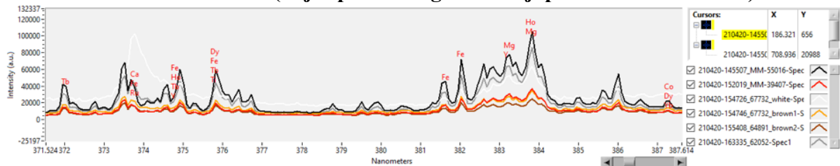
Tablica 7 Graf s rezultatima kvalitativne analize na različitim premazima helenističke keramike iz Ise (boja spektra odgovara boji premaza na keramici)
