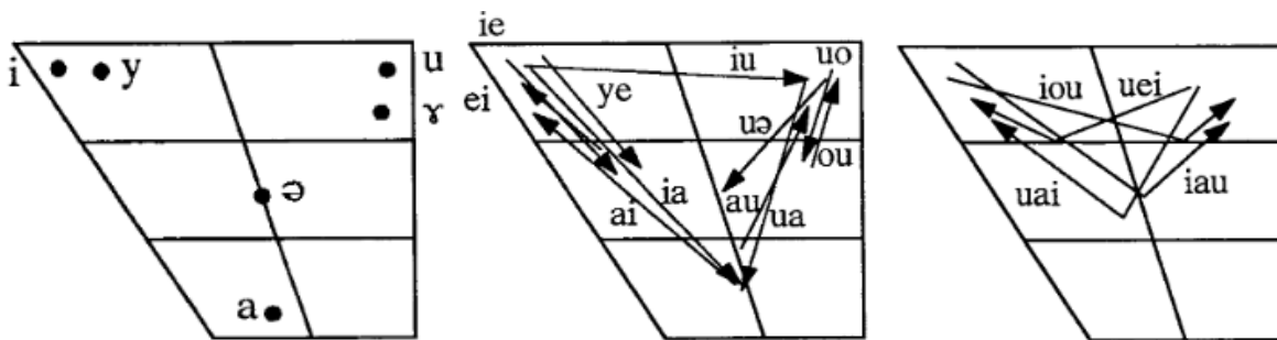
Slika 1: vokalski trapezoidi kineskih samoglasnika prema Lee i Zee (2003: 110)
