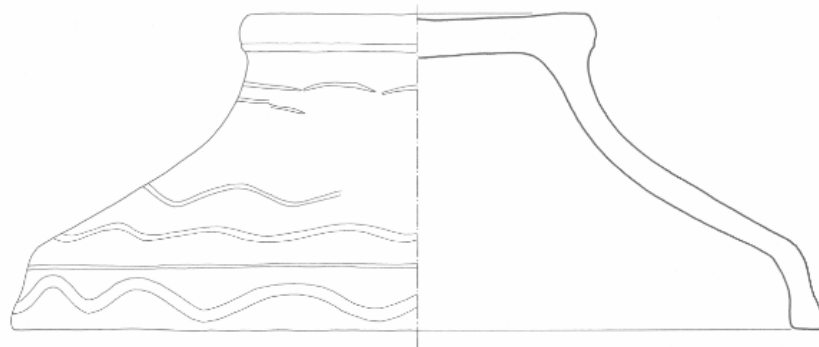
Slika 22 Rekonstruirani poklopac iz SJ 145 ukrašen valovnicama - svi crteži: terenska arheološka radionica Odsjeka za arheologiju u Bizovcu
