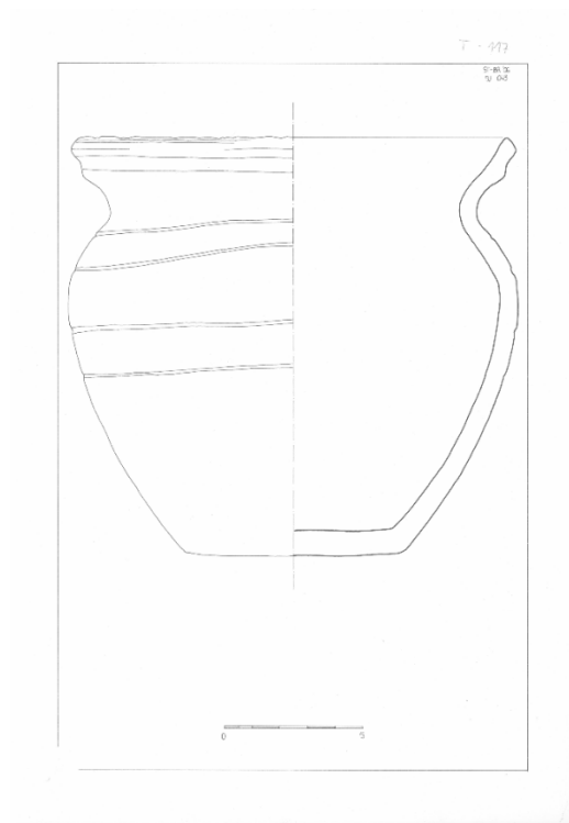
Slika 12 Ukrašeni lonac iz SJ 043 –svi crteži: terenska arheološka radionica Odsjeka za arheologiju u Bizovcu
