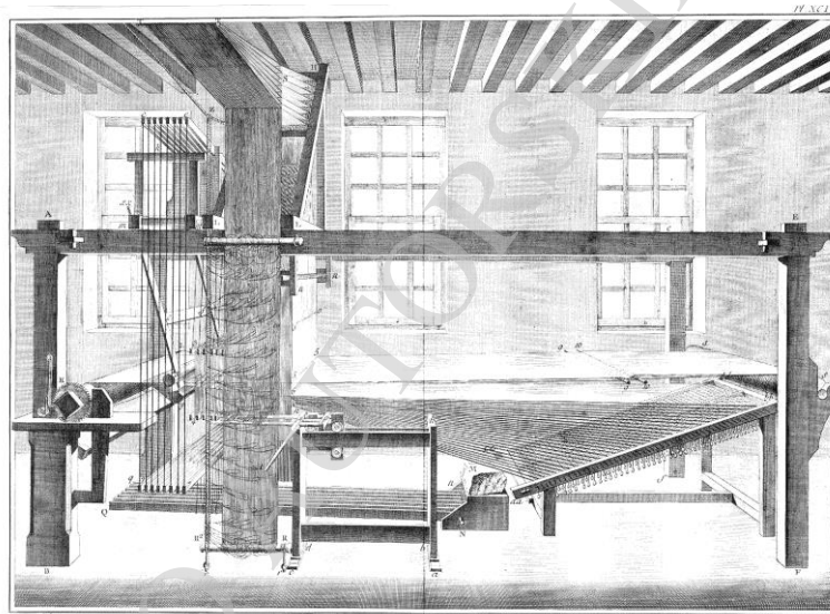
PLANCHE IV SOUTIC, Vue Perspective du Métier pour fabriquer le baršuna, vu dans l'endroit de la tête et du Drapeau des Têtes.
