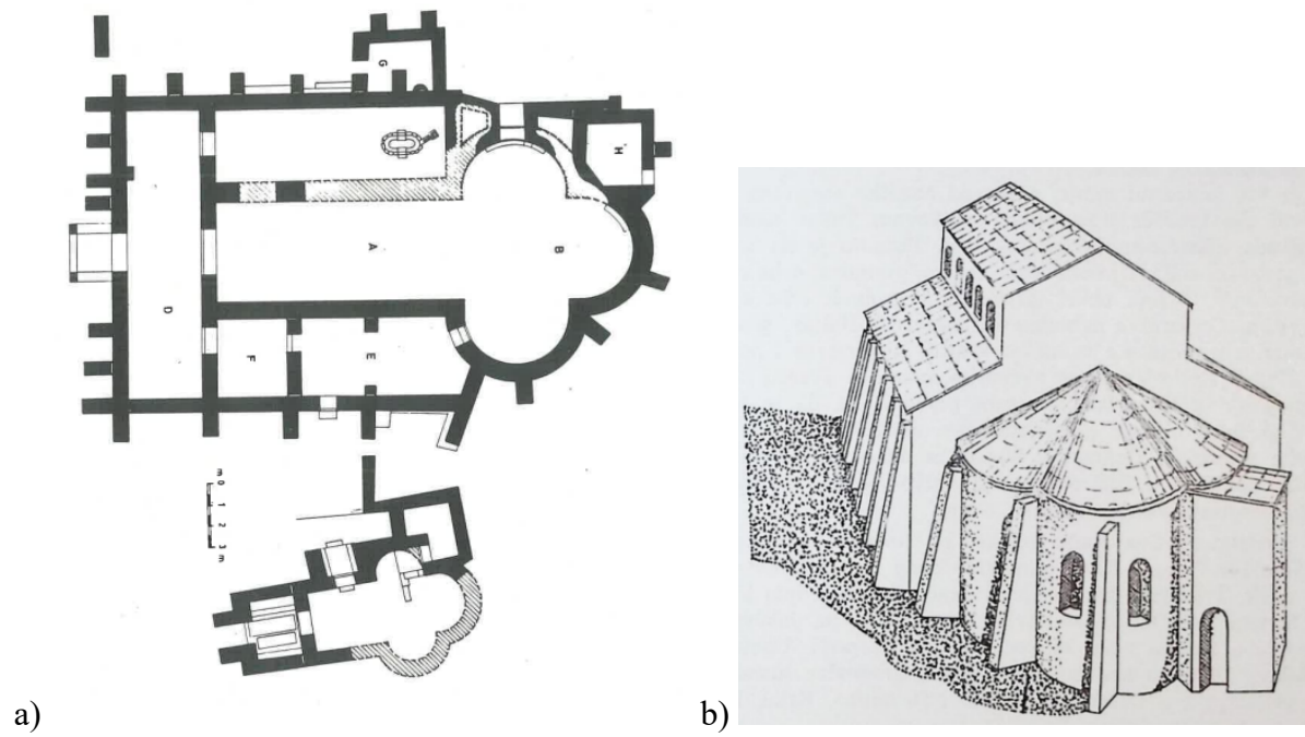
Slika 3: Crkva u Cimu, tlocrt (a) i rekonstrukcija (b)
