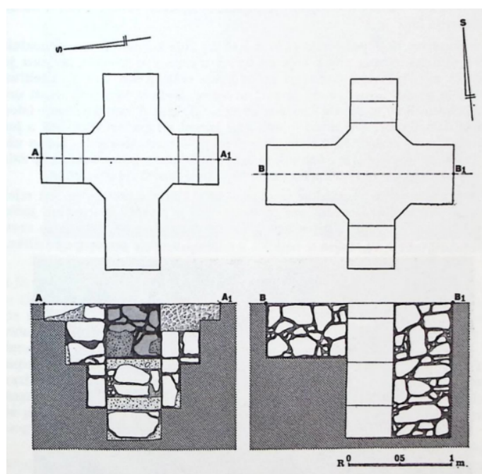
Slika 2: Krstionica u Barama, shema i presjek
