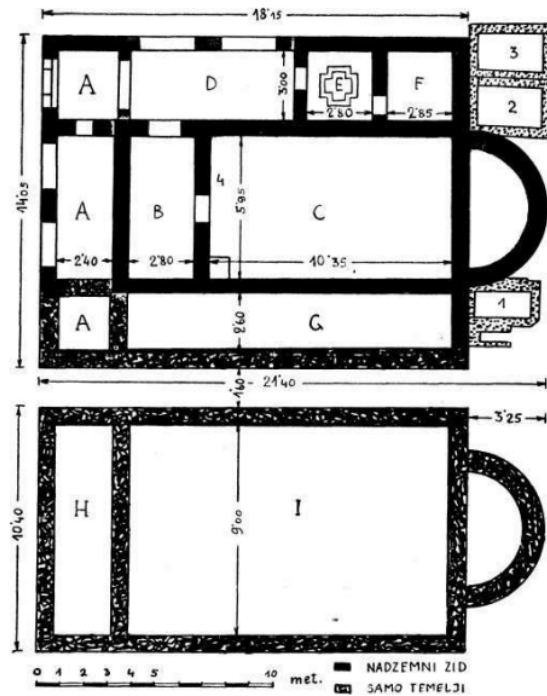
Slika 64: Tlocrt crkava na Mogorjelu
