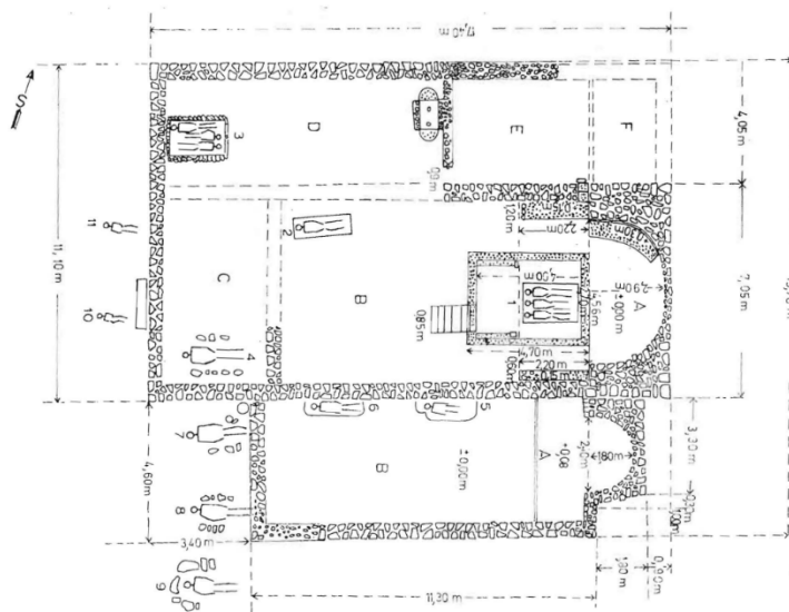
Slika 70: Tlocrt crkve u Gracu
