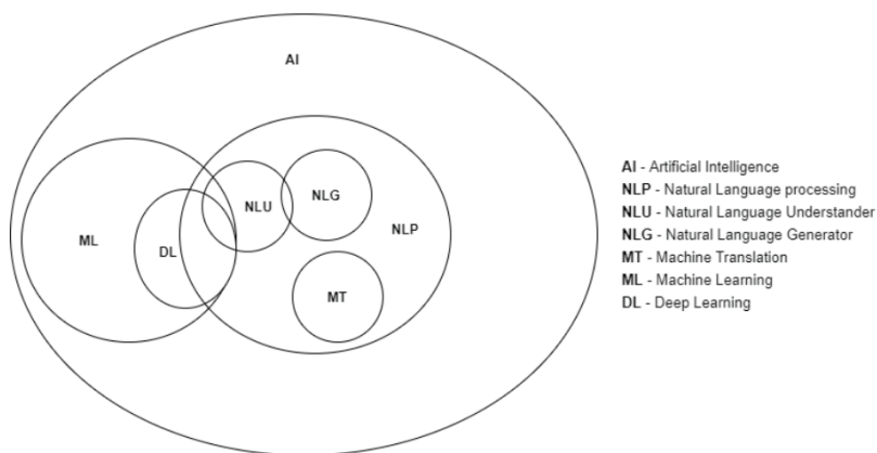
Slika 1. Područja vezana uz NLP i njihovi međusobni odnosi (Izvor: Šuman, 2021.)
