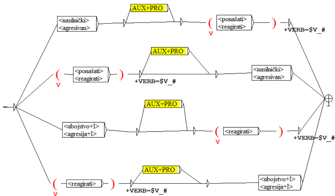
Slika 4. Sintaktička gramatika za glagole „ponašati“ i „reagirati“
