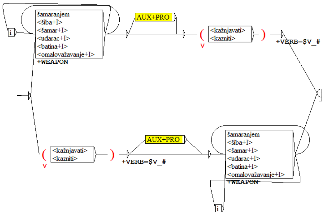
Slika 5. Sintaktička gramatika za glagole „kazniti“ i „kaznjavati“
