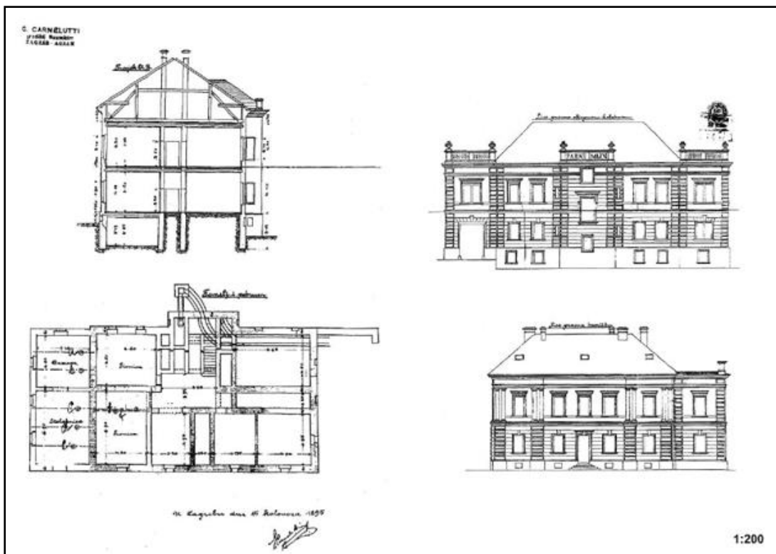
Sl. 8. G. Carnelutti, upravna zgrada, poprečni presjek a-b- i tlocrt temelja i podruma (lijevo); pročelje prema glavnom kolodvoru i dvorišno pročelje (desno), 1885. godine
