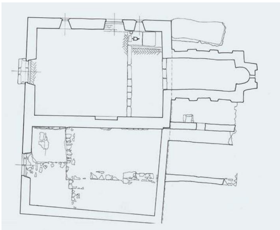
Slika 16. Tlocrt sv. Ivana kod Šilova sela. Izradila: Luciana Peko, vidi u: Željko Peković, Četiri elafitske crkve , 2008., str. 44.
