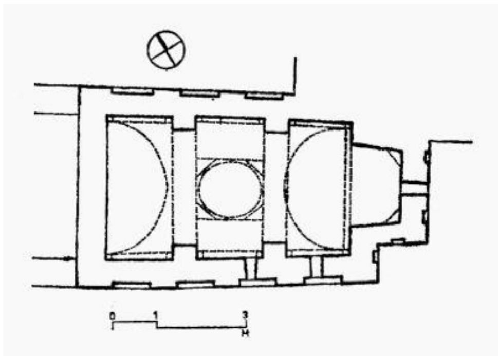
Slika 21. Rekonstrukcija tlocrta crkve sv. Mihajla u Pakljenjoj. Prema: Igor Fisković, vidi u: Tomislav Marasović, Dalmatia praeromanica , 4., 2013., str. 212.
