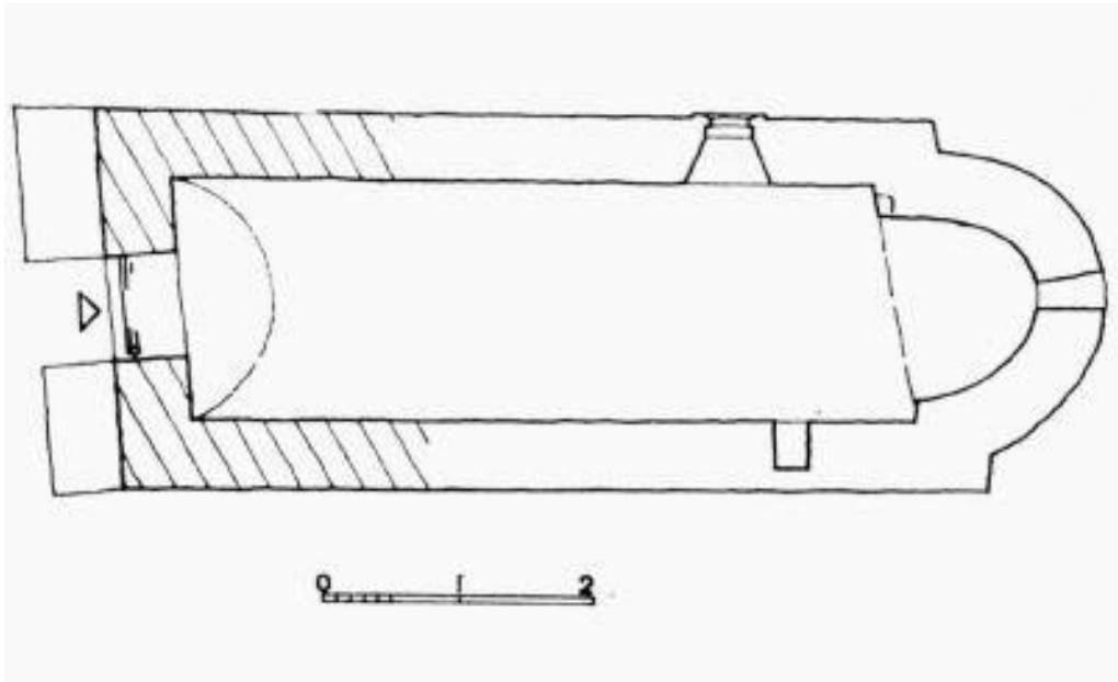
Slika 13. Tlocrt sv. Mihovila nad morem. Prema: I. Fisković, vidi u: Tomislav Marasović, Dalmatia praeromanica , 4., 2013., str. 205.
