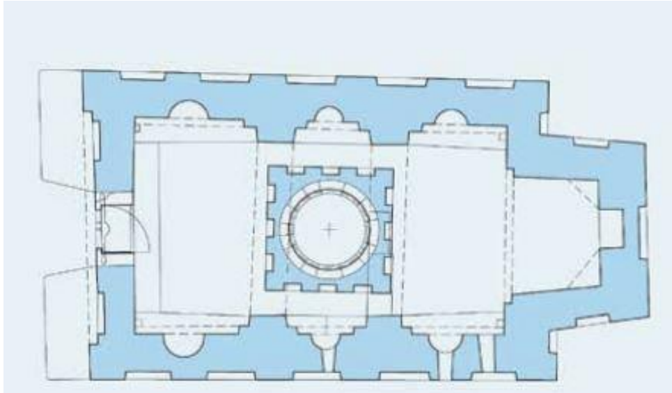
Slika 30. Tlocrt s položajem rekonstruirane kupole sv. Petra na Veljem Vrh. Prema: Željko Peković, vidi u: Željko Peković, Četiri elafitske crkve , 2008., str. 114.
