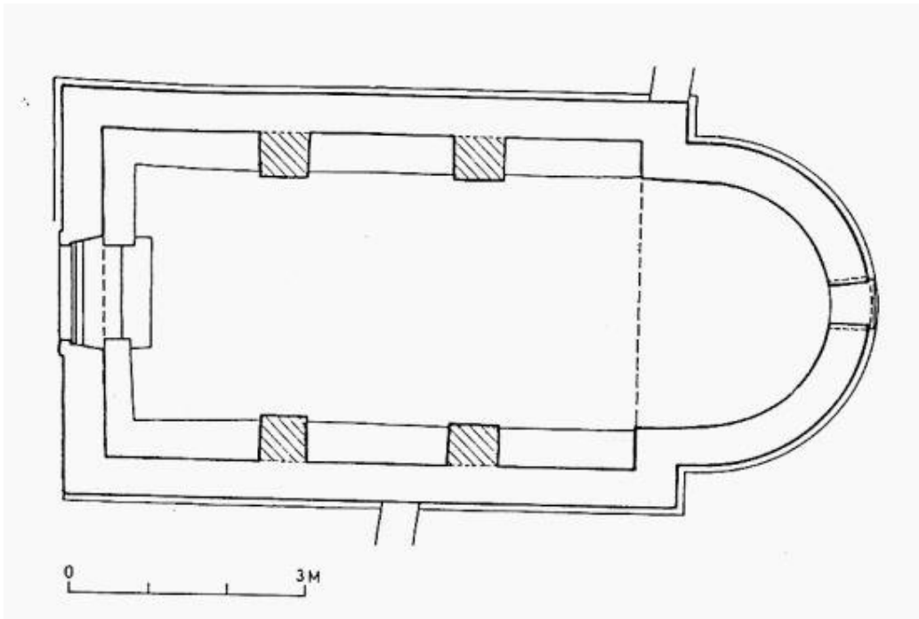
Slika 5. Tlocrt sv. Marije u Biskupiji. Prema: Igor Fisković, vidi u: Tomislav Marasović, Dalmatia praeromanica , 4., 2013., str. 208.
