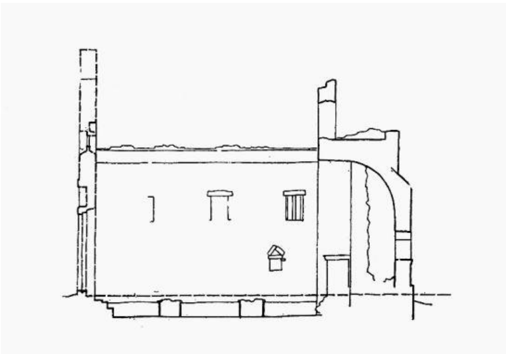
Slika 6. Uzdužni presjek crkve sv. Marije u Biskupiji. Prema: Igor Fisković, vidi u: Tomislav Marasović, Dalmatia praeromanica , 4., 2013., str. 208.
