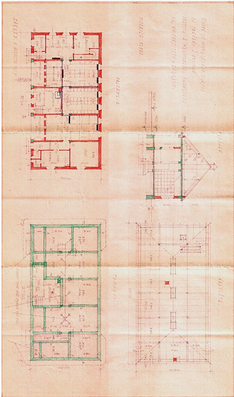
Nacrt 2, Temelj, prizemlje i krovšte gospodarske zgrade. (Izvor: HR – MEF – Opći spisi – Broj: 2714/1937. Predmet: Izgradnja štale za pokusne životinje. MINISTARSTVU PROSVJETE, opće odeljenje u/ BEOGRADU)
