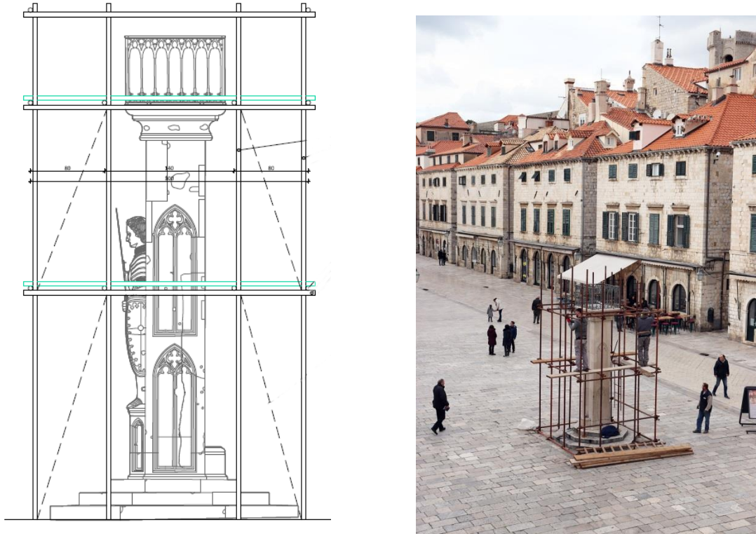
Slike 55, 56 . Zaštitna skela i njezino postavljanje
