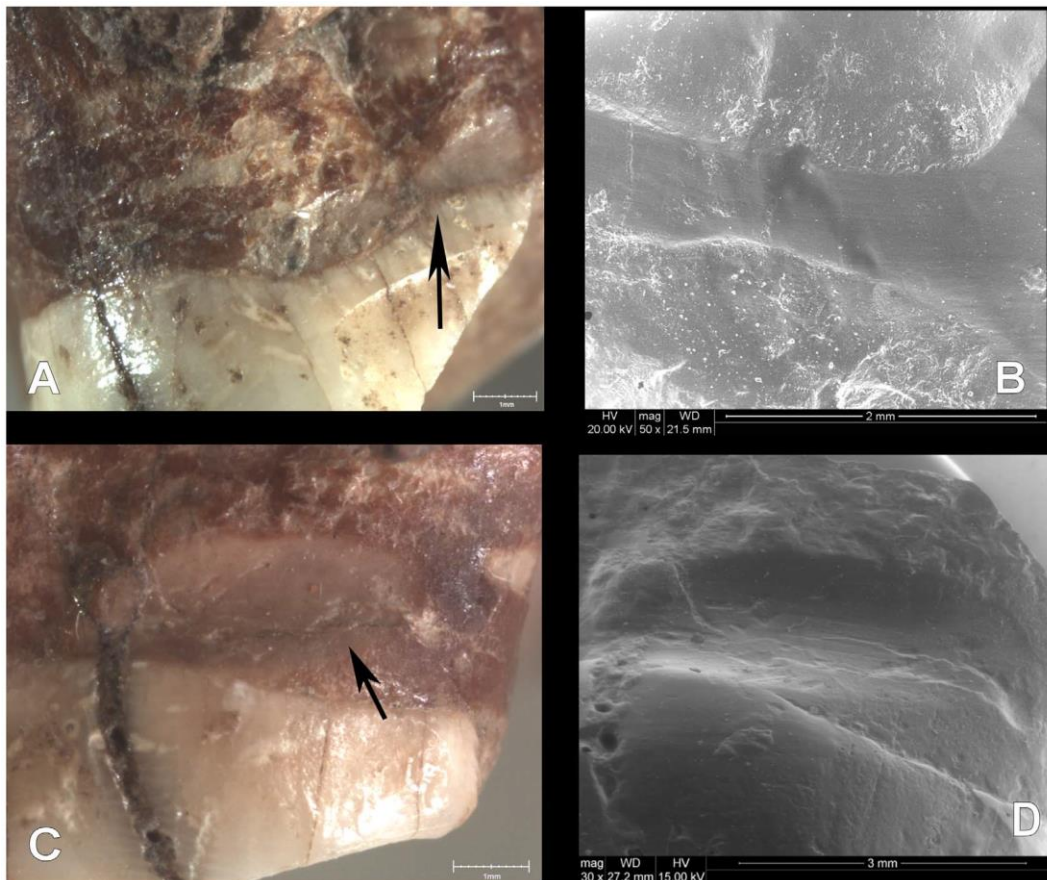
Slika 14. Inteprosimalni žljebovi na zubima neandertalaca s nalazišta Cova Forada (prema: Lozano et al. 2013: 4).
