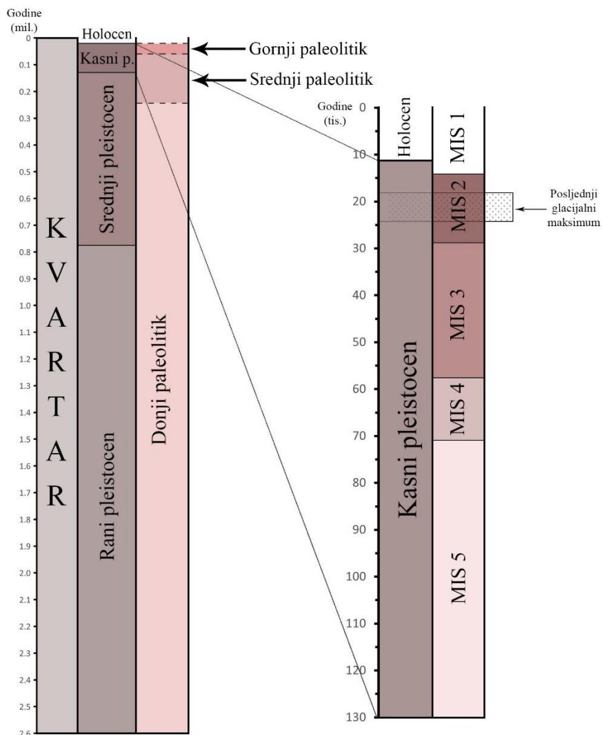
Tablica 1. Kronologija kvartara i kasnog pleistocena (izradila L. Vidas, prema: Lisiecki, Raymo 2005, Gibbard, Head 2010; http://struna.ihj.hr/naziv/kvartar/31729/#naziv ).
