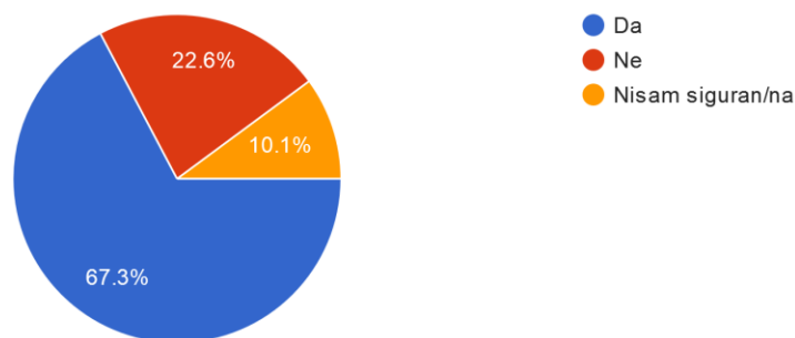
Graf 8: Omjer odgovora na deseto pitanje
