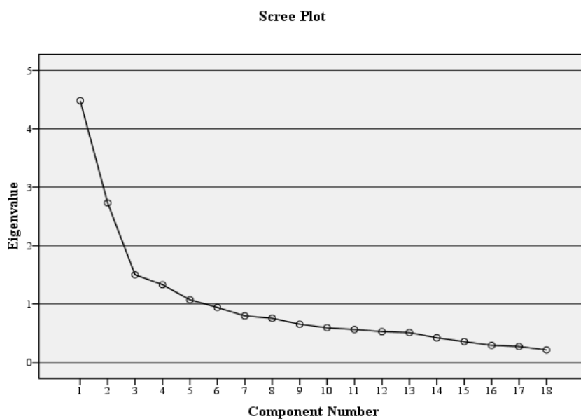
Grafikon 2. Svojstvene vrijednosti ( eigenvalue ) po pojedinim manifestnim varijablama Skale stavova o društvenim mrežama.
