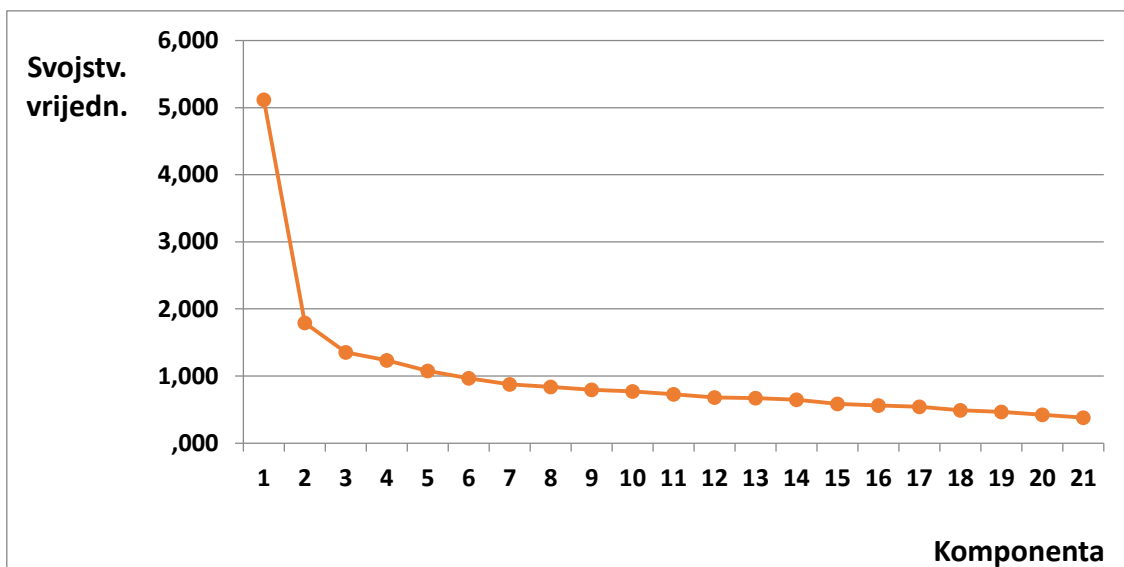
Grafikon 4. Svojstvene vrijednosti ( eigenvalue ) po pojedinim manifestnim varijablama Skale aktivnosti u slobodno vrijeme (N = 594)
