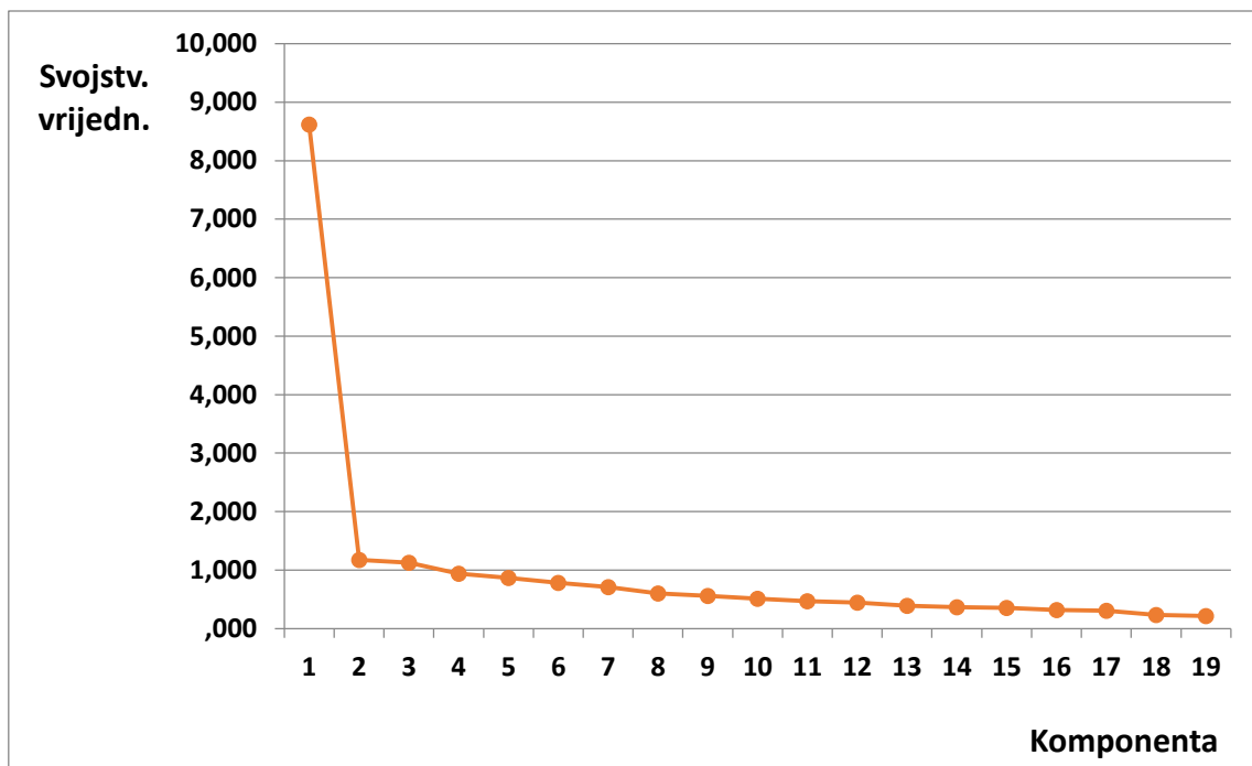
Grafikon 6. Svojev. vrijednosti ( eigenvalue ) po pojedinim manifestnim varijablama Skale kvalitete života (N = 594)
