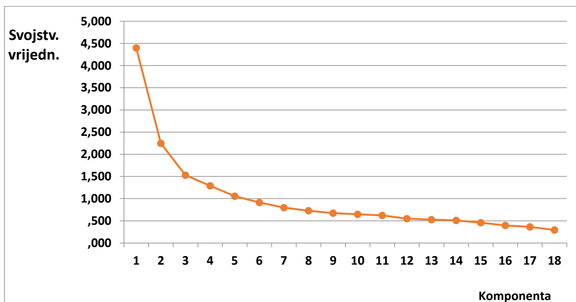
Grafikon 5. Svojstvene vrijednosti ( eigenvalue ) po pojedinim manifestnim varijablama Skale stavova o društvenim mrežama (N = 594)
