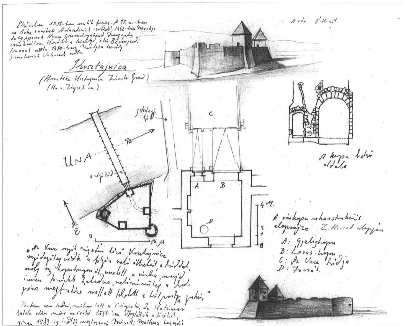
Nacrti utvrde Kostajnice na Uni (Frigyas König, 2016.)
