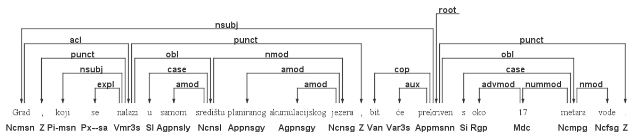
30. slika: Atributna rečenica iz UD-HR korpusa (Agić i Ljubešić 2015).
