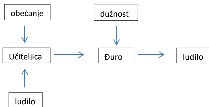
Slika 6. Aktantski model 3
