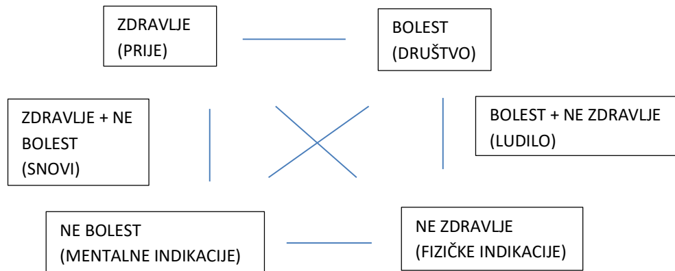
Slika 8. Semiotečki kvadrat
