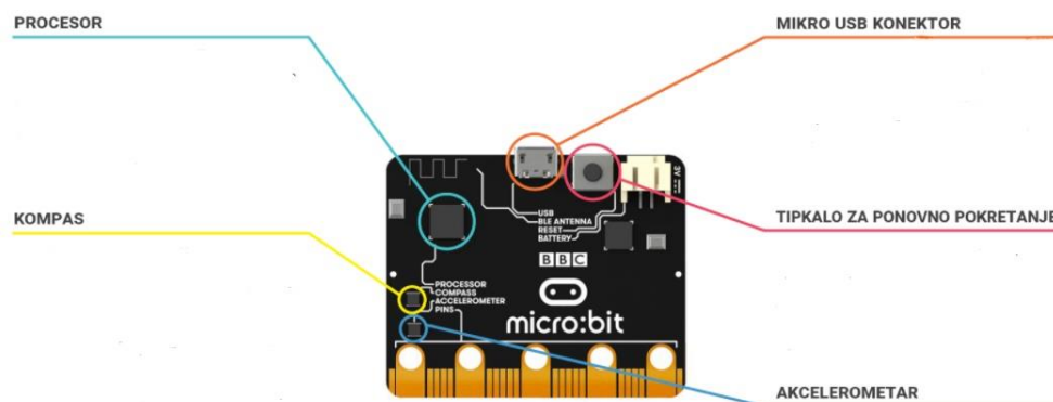
Slika 2. Prednja strana micro:bita
