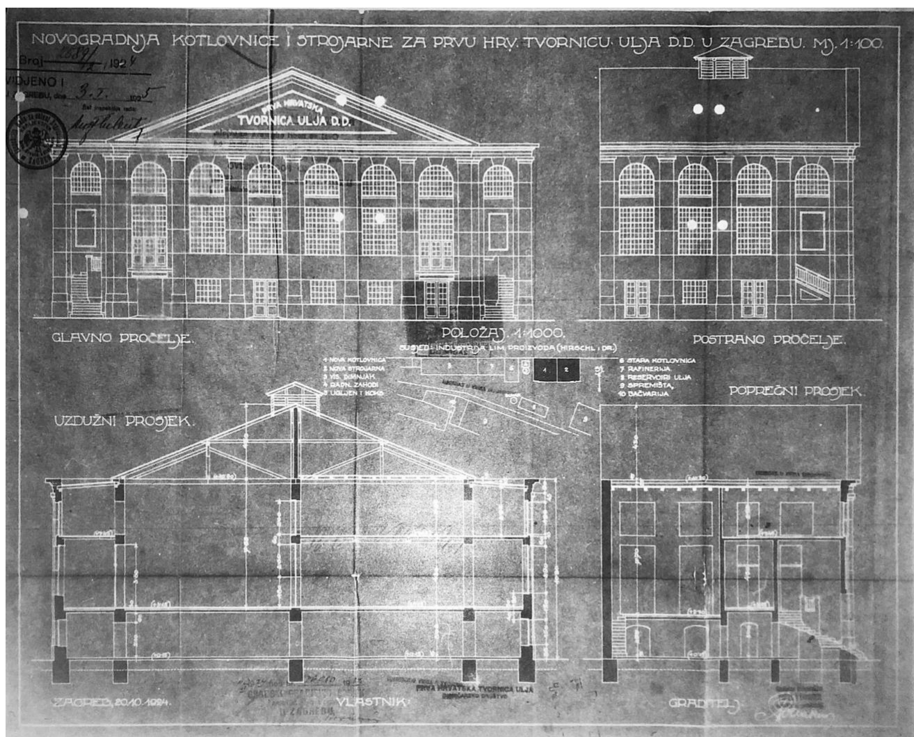
Slika 21. Nacrt glavnog pročelja i poprečnih, postranih i uzdužnih presjeka novogradnje kotlovnice i strojarne za Prvu hrvatsku tvornicu ulja d.d. u Zagrebu
