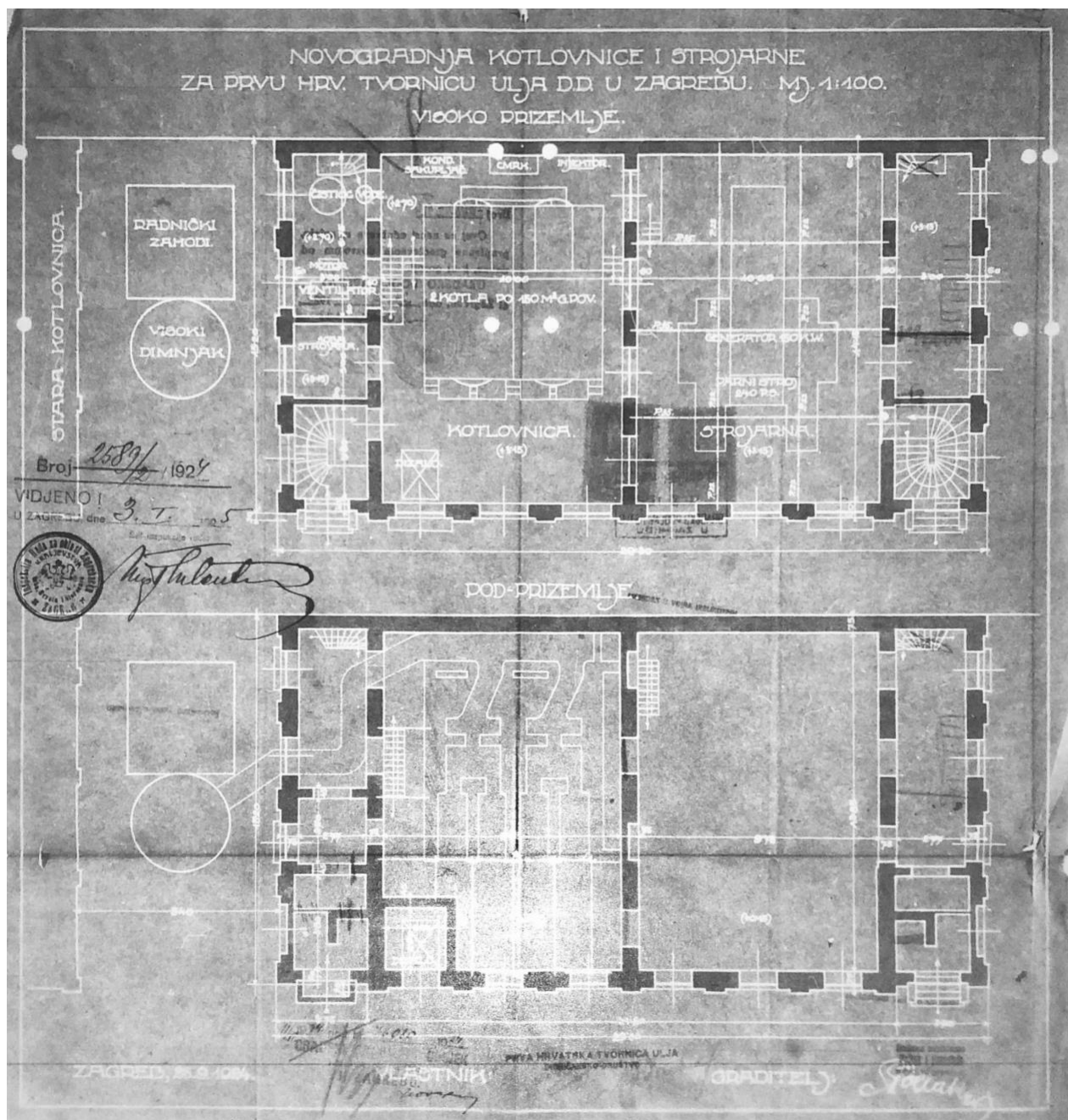
Slika 22. Nacrt tlocrta podrumskog prizemlja i visokog prizemlja novogradnje kotlovnice i strojarne za Prvu hrvatsku tvornicu ulja d.d. u Zagrebu
