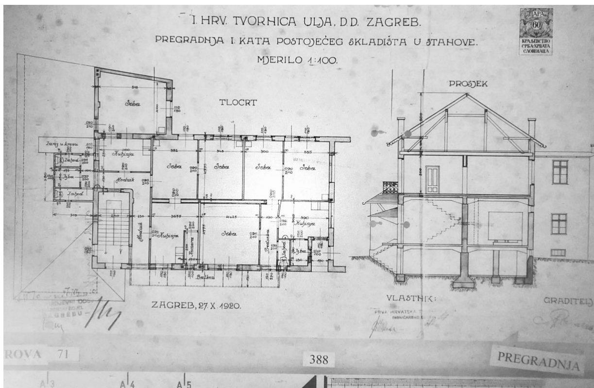
Slika 30. Nacrt za pregradnju prvog kata postojećeg skladišta u stanove
