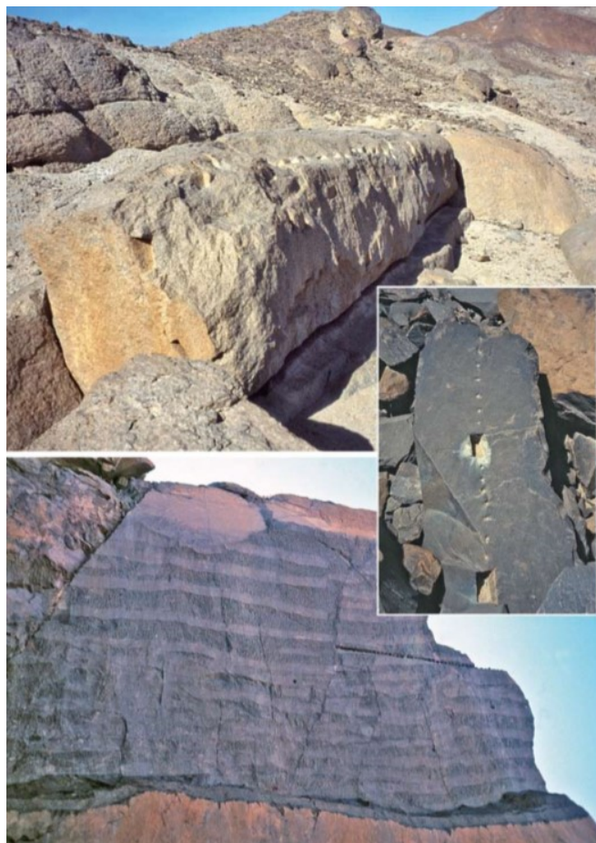
Slika 11 – Rimska tehnologija vađenja tvrdog kamena. Gore: napušteni stup u kamenolomu Mons Claudianus , još uvijek pričvršćen za stijenu, s tragovima rupa u obliku klinova i urezanim žlijebom duž donjeg ruba. Sredina: kameni blok u kamenolomu Wadi Hammamat, s rupama za klinove i pointillé rupama. Dolje: klesano lice porfirne stijene u kamenolomu Mons Porphyrites gdje su blokovi vađeni u više slojeva (Harrell – Storemyr 2009, 27, sl. 17)
