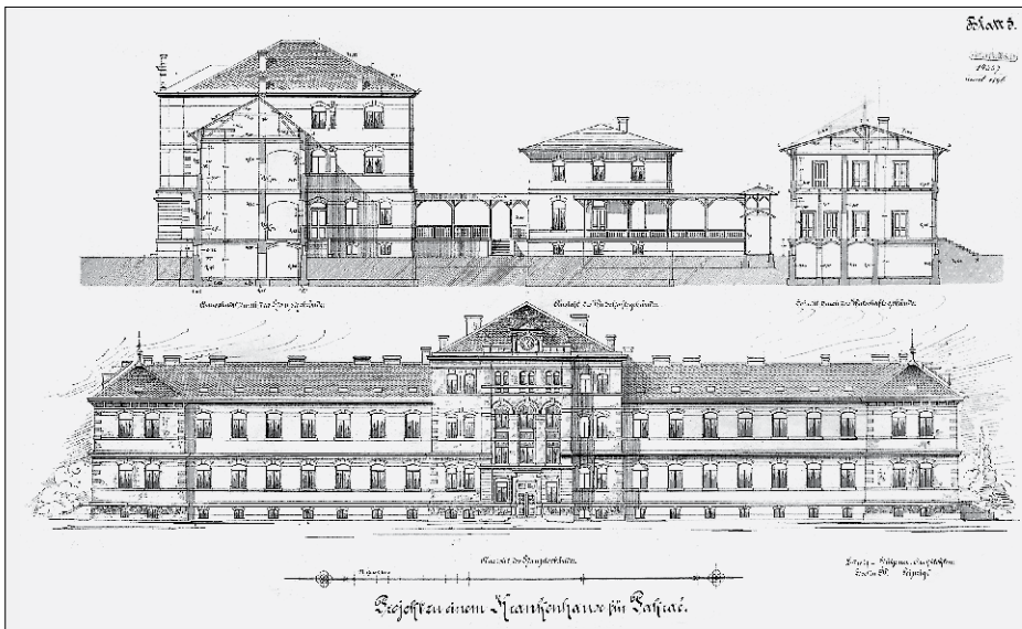
SL. 29. LUDWIG & HÜLSSNER: NEREALIZIRANI PROJEKT ZA SREĐNJU ZGRADU KRALJEVSKE ZEMALJSKE JAVNE BOLNICE U PAKRACU, 1894.
