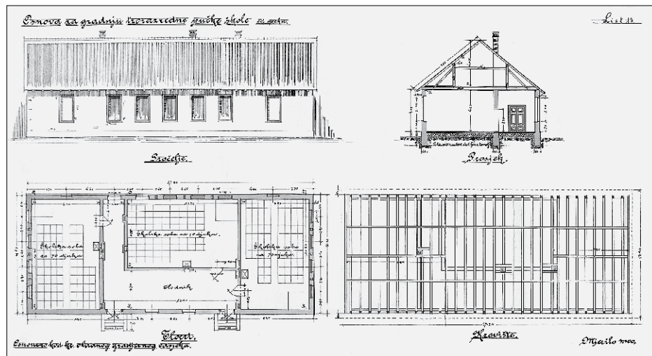
SL. 24. GRAĐEVNI ODSJEK ZEMALJSKE VLADE: TIPSKE PROJEKTI ZA IZGRADNJU TRORAZREDNE PUČKE ŠKOLE U HRVATSKOJ, 1895.
